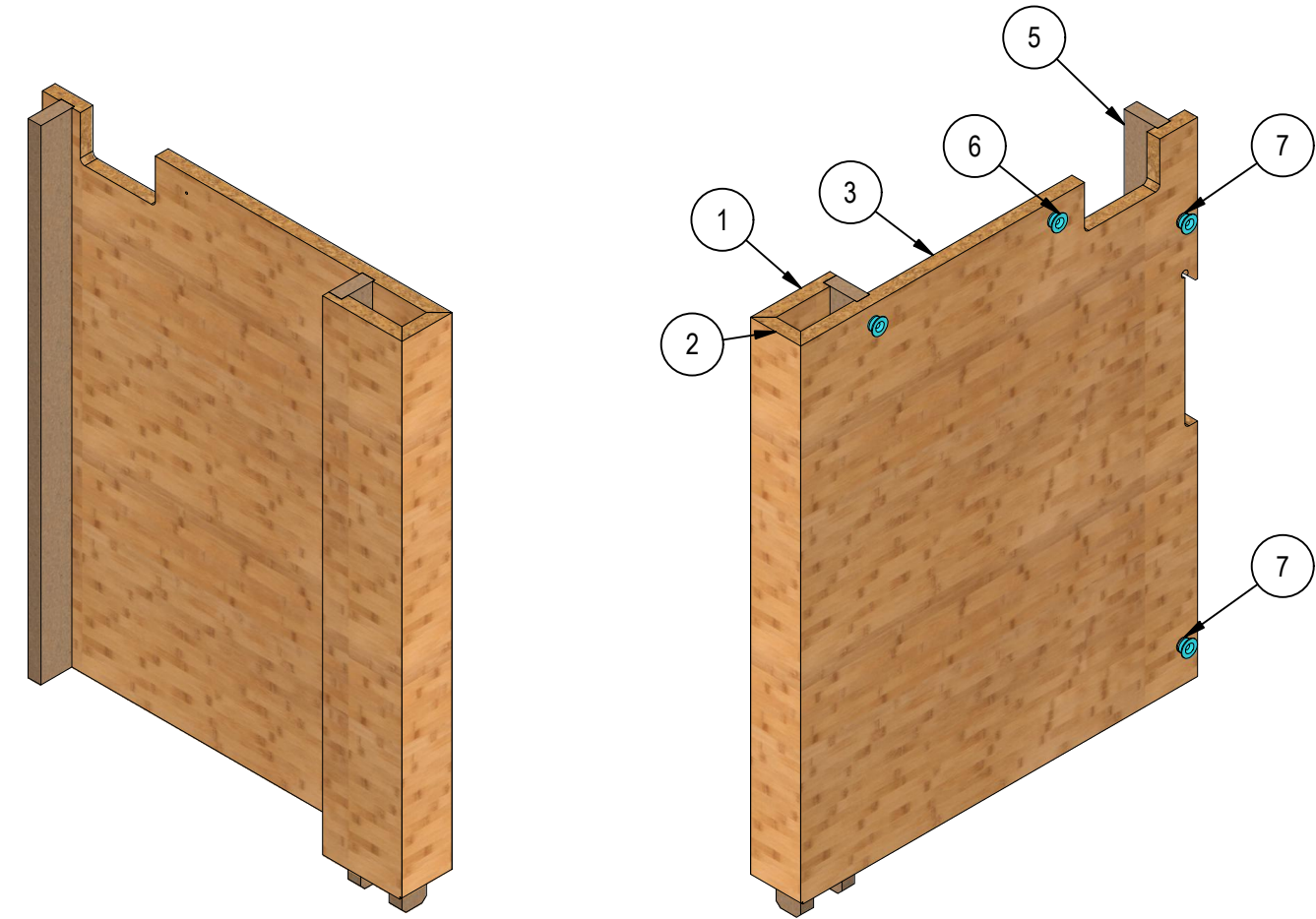
LEFT ISO SCALE 1/8
